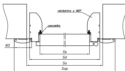
drzwi z ościeżnicą stałą
