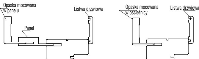
do drzwi CERBER II
