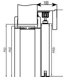
drzwi przesuwne – system naścienny z zabudową tunelową ZN
