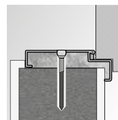
OPAL Montaż na dyble.
